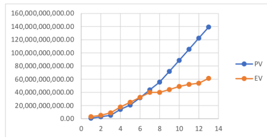
Gambar 6. Grafik perbandingan antara PV dan EV
