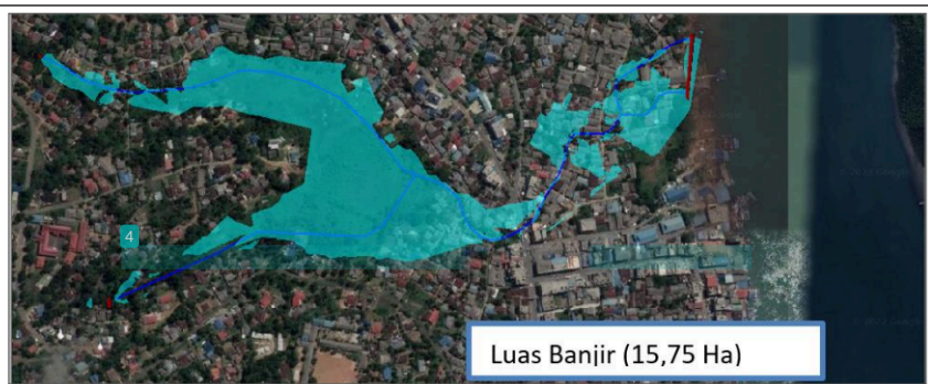
Gambar 11. Hasil pemodelan kondisi eksisting Q 25 tahun
