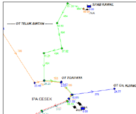
Gambar 4. Simulasi Epanet di Wilayah Pantai Kawal
