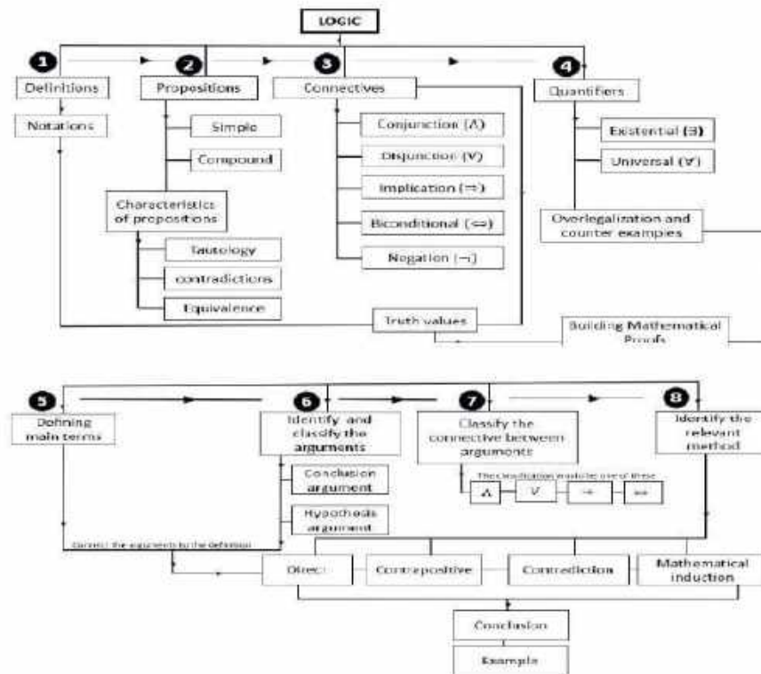
Gambar 1. Peta Konsep Logika dan Bukti Matematis (Issa & Majuma, 2019)
