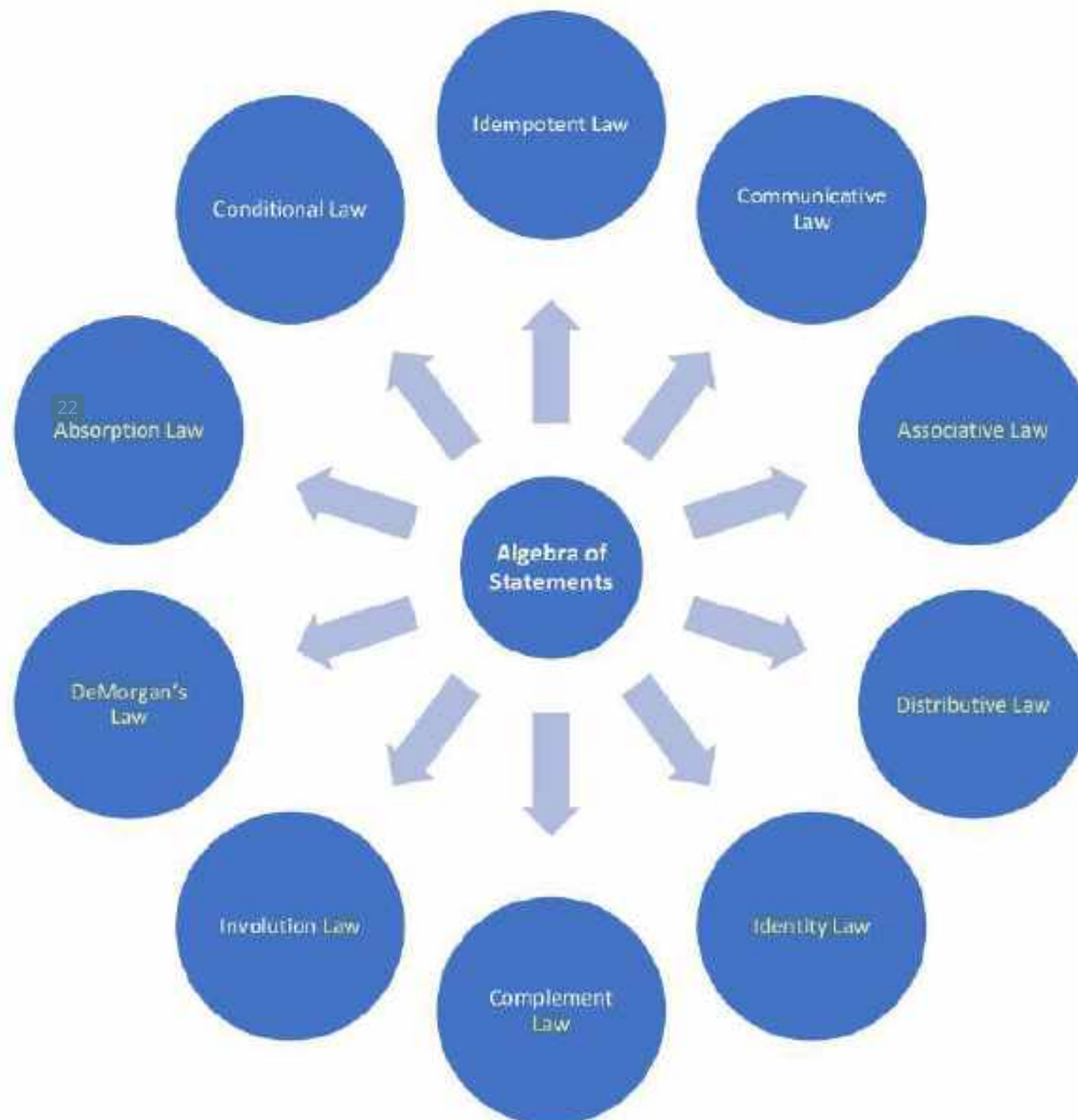
Gambar 9.1 Peta konsep aljabar pernyataan
